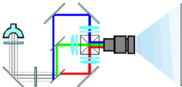
Obr.1 Technologie zobrazování LCD
