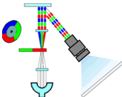
Obr.2 Technologie zobrazování DLP
