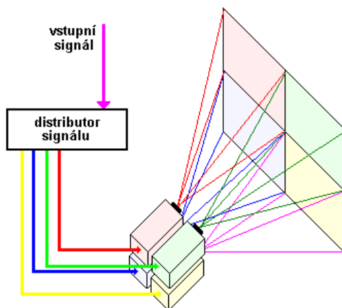
Obr.1 Princip sekvenčního zobrazování
